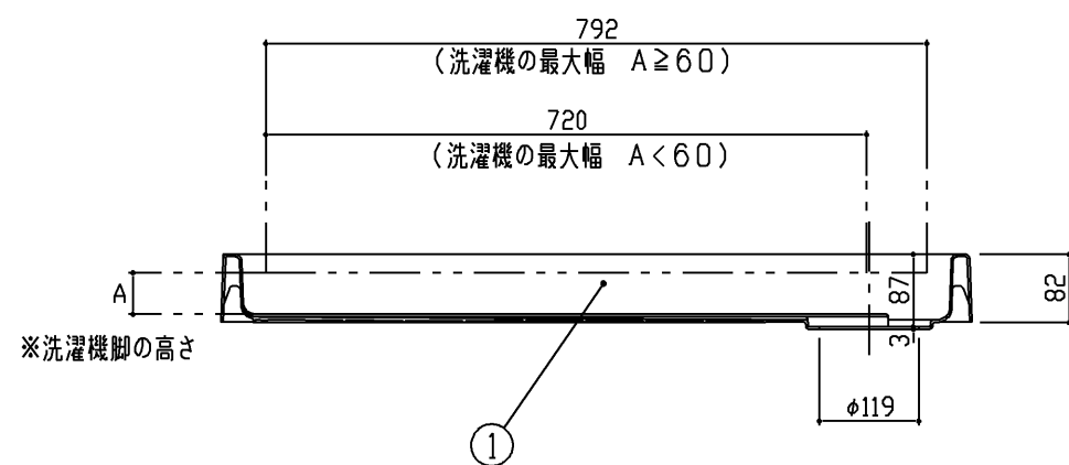
断面A-A
